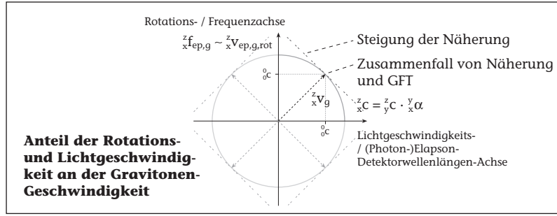
Abbildung 4.2: Die Darstellung zeigt, unter welchen Bedingungen das Pound-Rebka-Snyder-Experiment mit der GFT zusammenfällt. Der Gravitonen-Geschwindigkeitsvektor – am Kreismittelpunkt ansetzend – stellt die Geschwindigkeitseigenschaft der Oberfläche eines Elapsonen-Zylinders dar.
