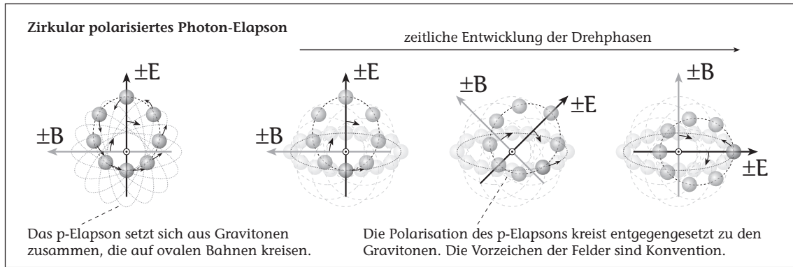
Abbildung 5.3: Ein zirkular polarisiertes Photon-Elapson ( p -Elapson) ist aus Gravitonen aufgebaut, die auf zueinander im Winkel stehenden, elliptischen Bahnen um sein Zentrum kreisen. Das p -Elapson rotiert mit der gleichen Frequenz wie die Gravitonen – in entgegengesetzter Richtung –, die der Frequenz eines unpolarisierten Elapsons gleicher Gravitonen-Anzahl entspricht. Die Polarisation erzeugt eine zirkular schwingende Abstrahlung von Gravitonen-Dichtedifferenzen in die Raumzeit, die seinem elektromagnetischen Feld entspricht. Die Vorzeichen der Felder sind dabei Konvention und es ist noch nicht klar, in welcher Orientierung diese zur gültigen Konventionen stehen.
