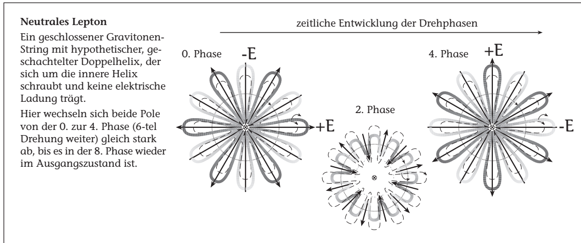
Abbildung 5.7: Die Grafik zeigt eine hypothetische Struktur eines elektrisch neutralen Leptons mit n_{pol} = \frac{n_{wel}}{n_{polwel}} = \frac{12}{2} = 6 (Berechnungen im Anhang 14.2, Seite 166). Die Gravitonen eines Gravitonen-Strings mit wechselnder Gravitonen-Dichte bewegen sich auf einer doppelt geschachtelten, helixförmigen Spiralbahn um ein gemeinsames Rotationszentrum. In der gezeigten Struktur blinkt das Lepton mit der De-Broglie-Frequenz in einem Wechsel zwischen einer positiven und negativen Polarisierung und damit elektrischen Ladung. Aus weitem Blickwinkel erscheint das Lepton vornehmlich elektrisch neutral, während von nahem Blickwinkel die differenzierte Polarisierung in ihrer zeitlichen Dynamik die elektroschwache Wechselwirkung erzeugt.
