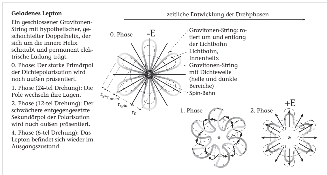
Abbildung 5.6: Die Grafik zeigt eine hypothetische Struktur eines elektrisch geladenen Leptons mit n_{pol} = \frac{n_{wel}}{n_{polwel}} = \frac{6}{1} = 6 (Berechnungen im Anhang 14.2, Seite 166). Die Gravitonen eines Gravitonen-Strings mit wechselnder Gravitonen-Dichte bewegen sich auf einer doppelt geschachtelten, helixförmigen Spiralbahn um ein gemeinsames Rotationszentrum. In der gezeigten Struktur blinkt das Lepton mit der De-Broglie-Frequenz in einem Wechsel zwischen einer leicht positiven und einer stärker negativen Polarisierung und damit elektrischen Ladung. Aus weitem Blickwinkel erscheint das Lepton vornehmlich elektrisch negativ geladen, während von nahem Blickwinkel die differenzierte Polarisierung in ihrer zeitlichen Dynamik die elektroschwache Wechselwirkung erzeugt. Der Normradius r_0 ist dabei die Bezugseinheit mit r_0 = \frac{\hbar}{m_{lep} \cdot c} .
