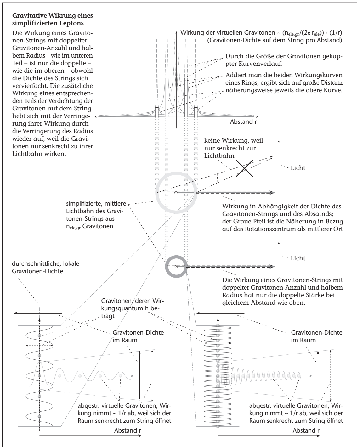
Abbildung 13.2: Die Grafik beschreibt die gravitative Wirkung anhand eines simplifizierten Gravitonen-Strings des Leptons. Unter der Annahme des Struktur-Postulats, dass jedes Graviton ein Wirkungsquantum h ist, und unter Vernachlässigung des Vakuums ergibt sich auf großer Distanz die Formel von Einstein. Die Wirkung der abgestrahlten, virtuellen Gravitonen nimmt mit \frac{h}{r} bezüglich des Abstandes r zum String ab und nicht(!) mit \frac{h}{r^2} , weil entlang des Strings die virtuellen Gravitonen immer wieder neu erzeugt werden. Die Wirkung eines Gravitons kann aufgrund seiner Ausdehnung nicht ins Unendliche steigen, sondern wird gekappt. (Die Ausdehnung der Gravitonen in die Fundierung übernehmen!)
