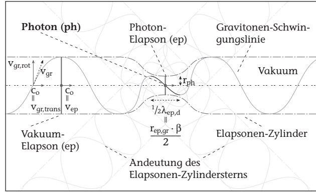
Abbildung 5.1: (Bildbeschriftung überarbeiten.) Darstellung des u-n-Elapsons als Einschnürung in einem Elapsonen-Zylinder mit der dazugehörigen Graviten-Schwingungslinie. Die Graviten-Schwingungslinie symbolisiert die Schwingungseigenschaften der Graviten bzw. der Elapsonen-Zylinderoberfläche. Als u-n-Elapson wird das gesamte, durch das erzeugende Elapson entfachte Raumzeit-Phänomen bezeichnet.
